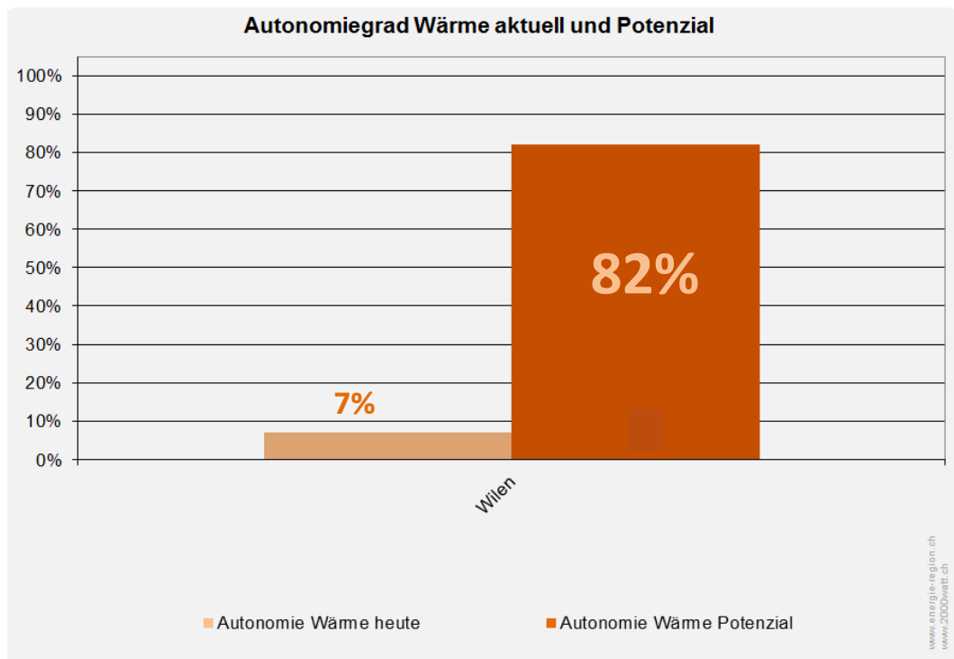
Abbildung 17: Potenziale für Wärmeautonomie bei heutigem Verbrauch.
